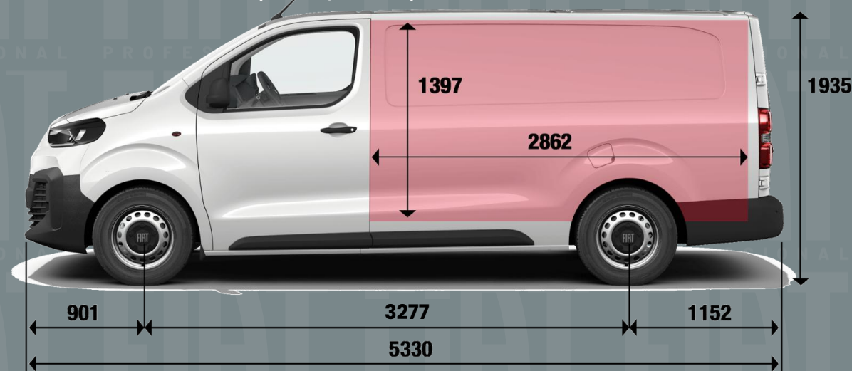
SCUDO L3 (6,1m³ / 6,6m³)
