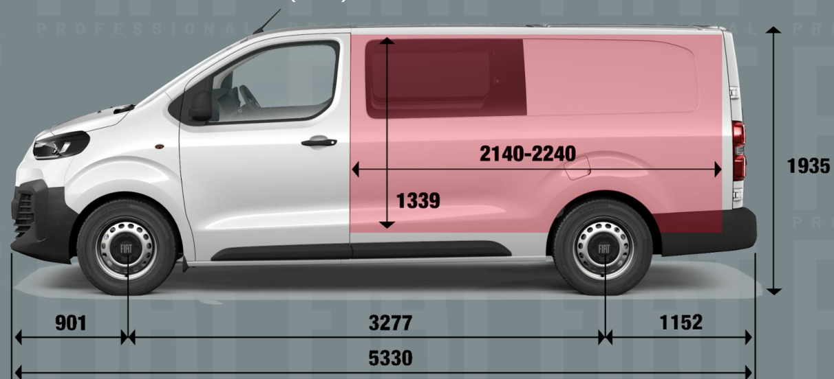
SCUDO CREW VAN L3 (4m³)
