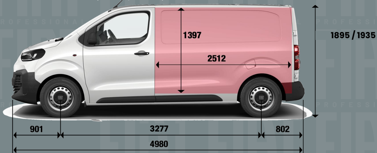
SCUDO L2 (5,3m³ / 5,8m³)
