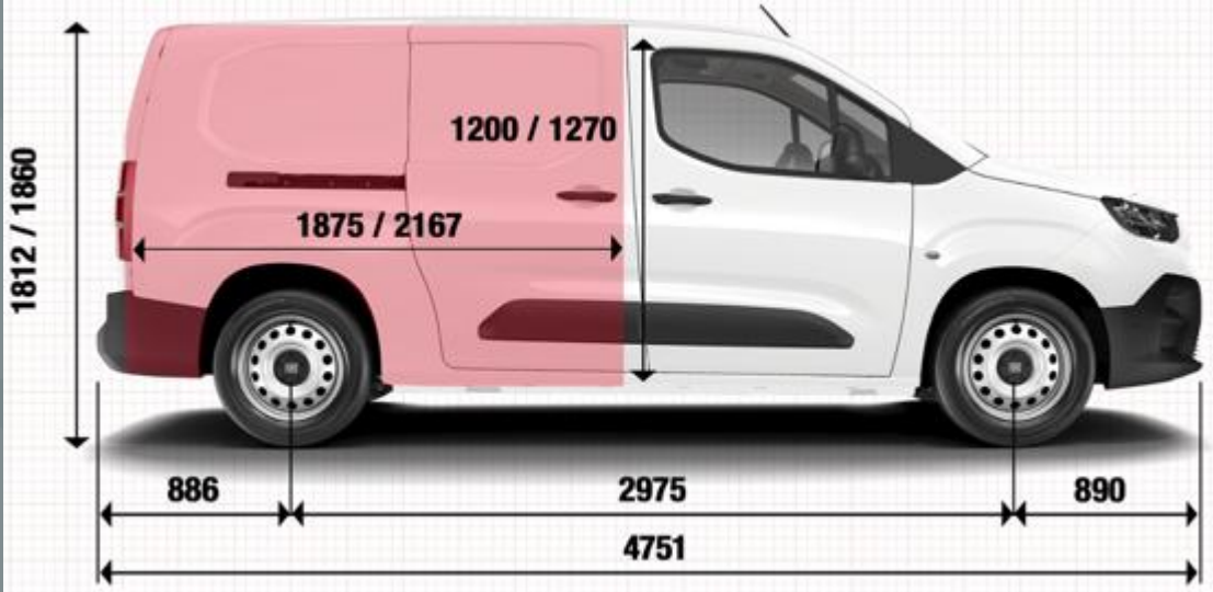
DOBLÒ L2 (3,9m³ / 4,4m³)
