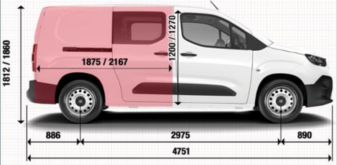
DOBLÒ CREW VAN L2 (1,8m³ / 3,5m³ / 4,0m³)
